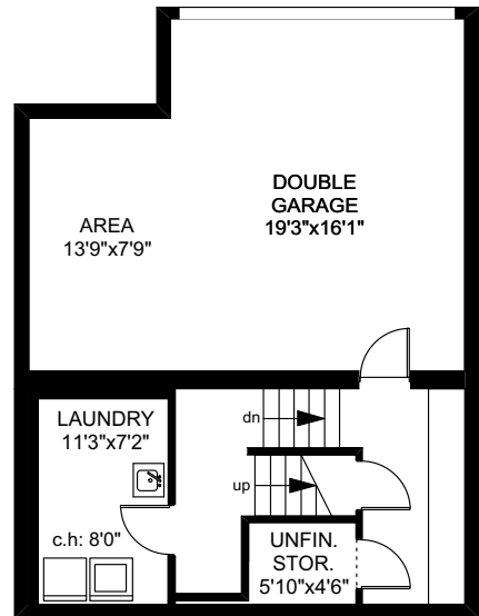
BASEMENT 331 SQ.FT
